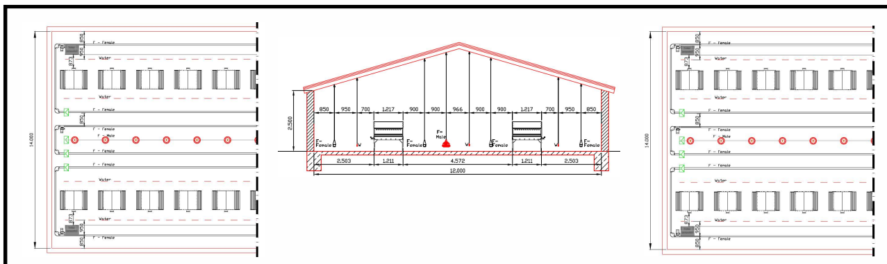
ESQUEMA DE UNA NAVE DE REPRODUCCION 12m Y 14m.
